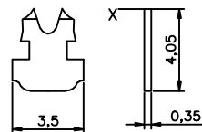
平面二叉标准端子
