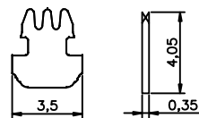
平面三爪端子
